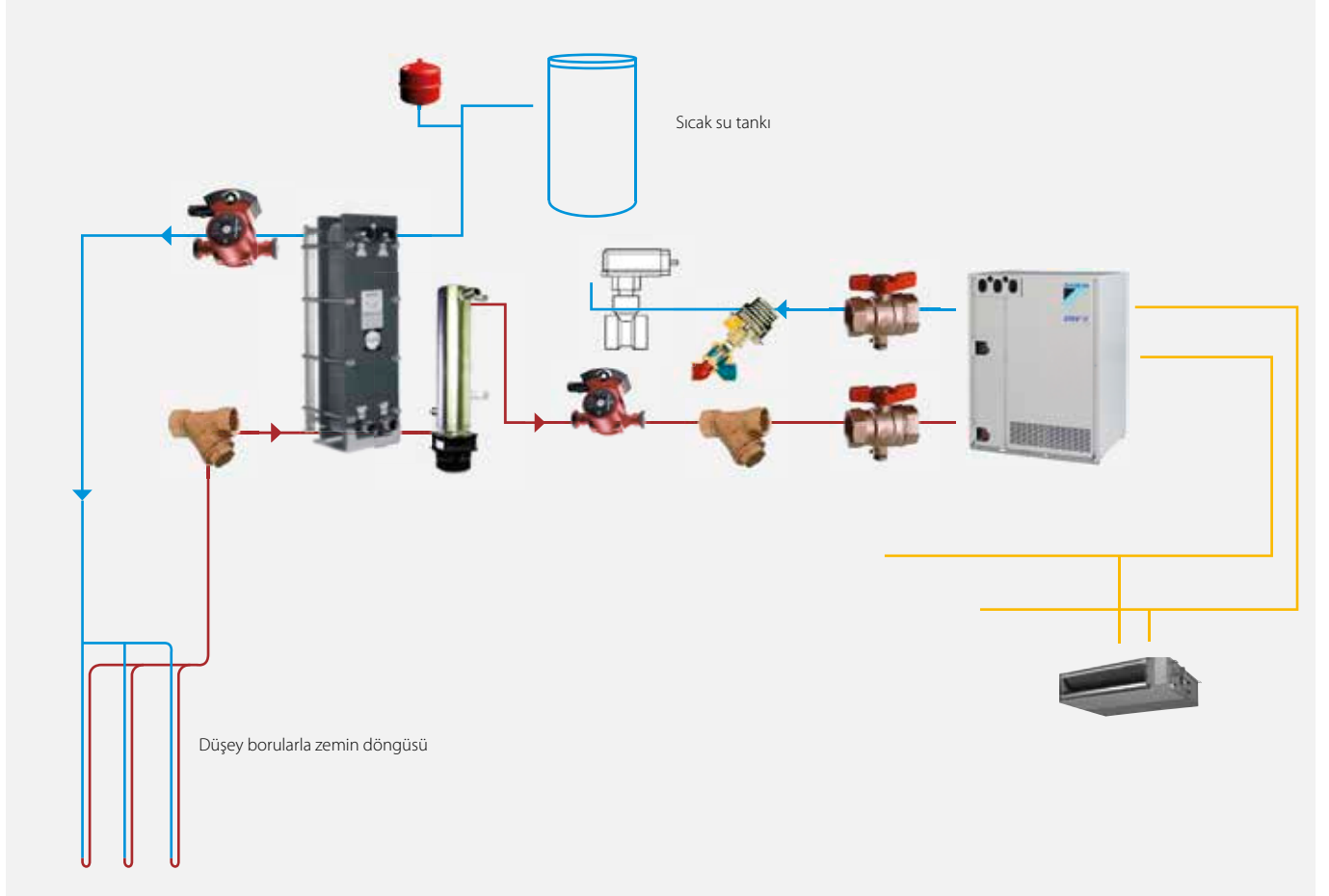
Genleşme tankı
